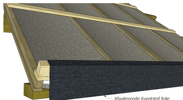
Figuur 7 - Afwaterende kunststof folie
