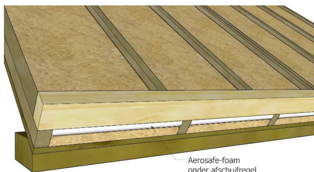
Figuur 4 - Aerosafe-foam onder afschuifregel
