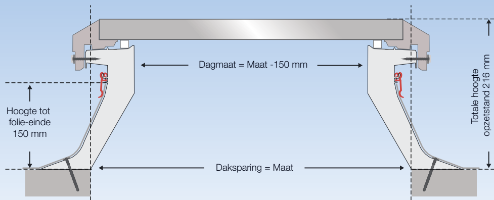
VlakGlasraam met PVC-opstand van 150 mm.
