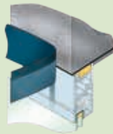
Cladseal EXT voorzien van machinaal aangebrachte zelfklevende strip, één- of tweezijdig Cladseal SA-Fix
