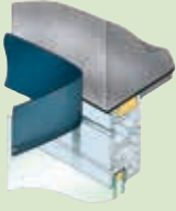
Cladseal EXT mechanisch bevestigd in het raamprofiel met een aangelast rubberprofiel Cladseal P-Fix
